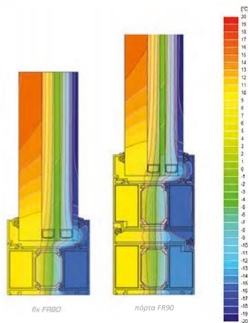
παράδειγμα ισοθερμικής κατανομής για το συνδυασμό πλαισίου και φύλλου παραθύρων στο σύστημα FR90
