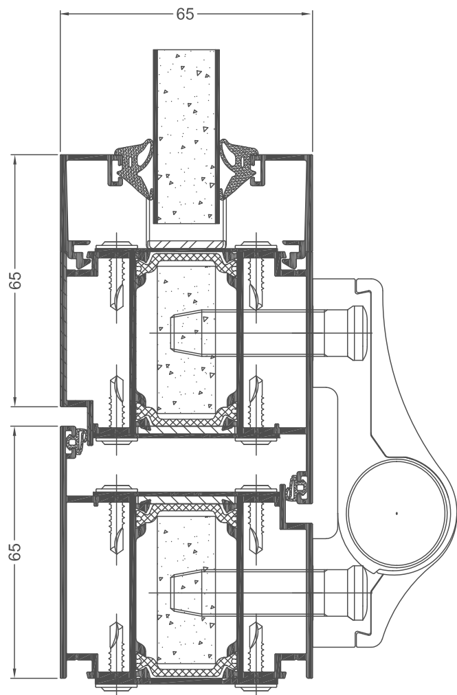
FR65 door cross section (FR024 + FR024)
